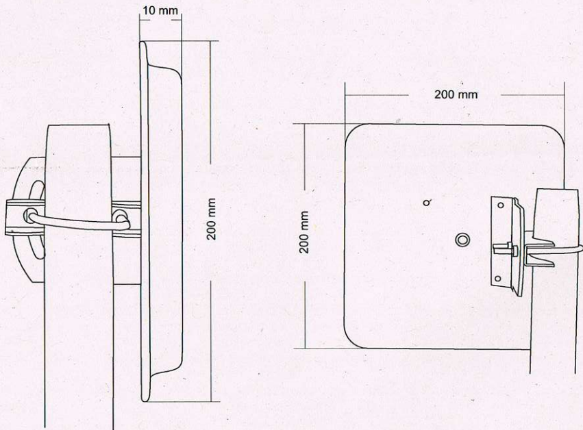
Przykład pozycjonowania anteny pod różnym kątem.
